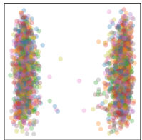
Layer 6
