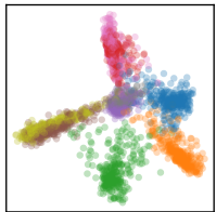
Layer 18
