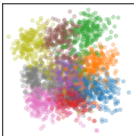
Layer 13
