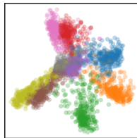
Layer 20
