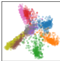
Layer 21
