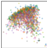
Layer 9
