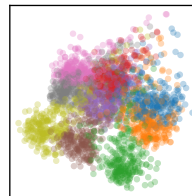
Layer 16
