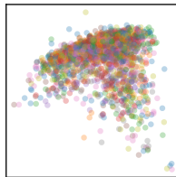
Layer 8
