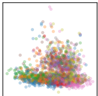
Layer 12
