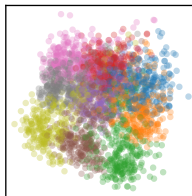
Layer 15
