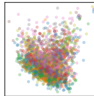
Layer 10
