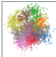
Layer 14
