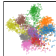
Layer 17
