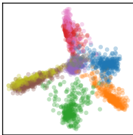
Layer 19
