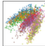
Layer 11
