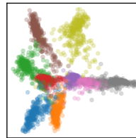
Layer 22
