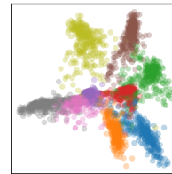
Layer 23
